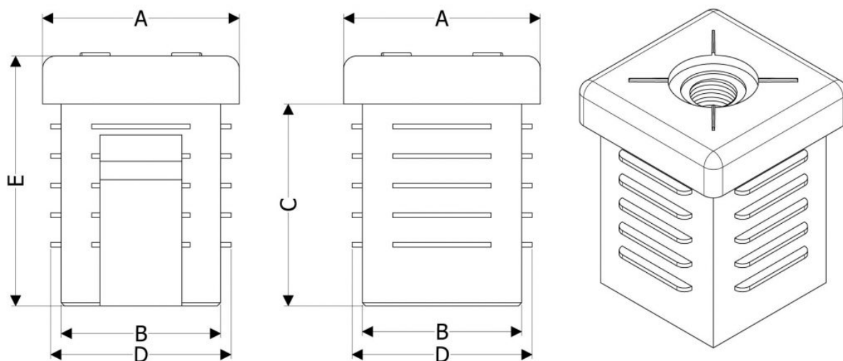
Wymiary wkładki z gwintem M10
